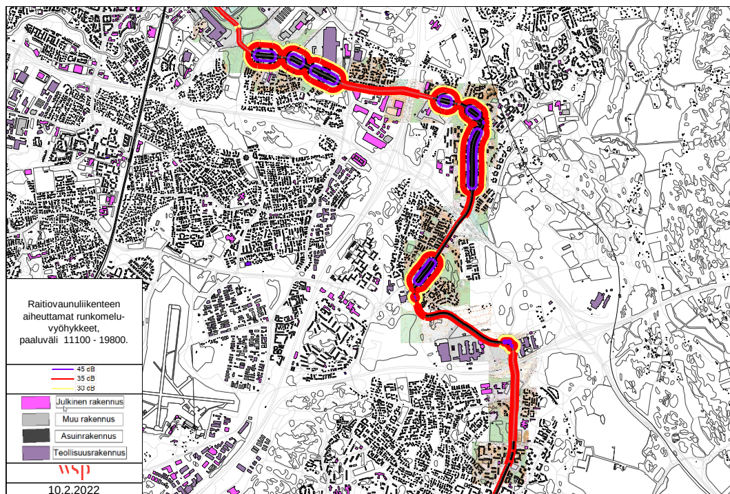
Kuva 5. Raitiovaunuliikenteen aiheuttamat runkomelualueet raitiotien itäisellä puoliskolla.
