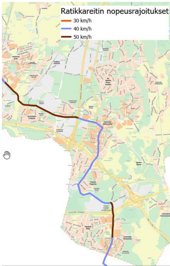
Kuva 2. Raitiotieosuuksien nopeusrajoitukset raitiotielinjauksen itäisellä puoliskolla.
