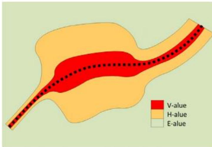
Kuva 3. Havainnekuva radan ympäristön värähtelyalueista (VTT 2014).
