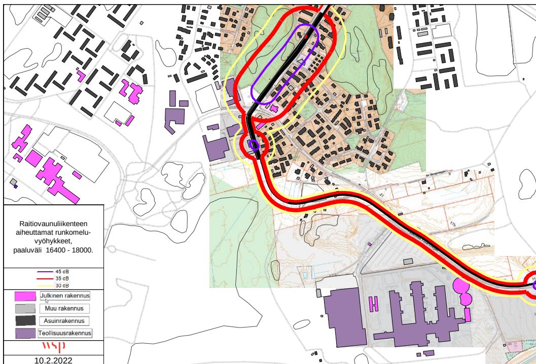
Kuva 9. Raitiovaunuliikenteen aiheuttamat runkomelualueet Vaaralan ja Kuussillan alueilla, paaluväli 16400 - 18000.
