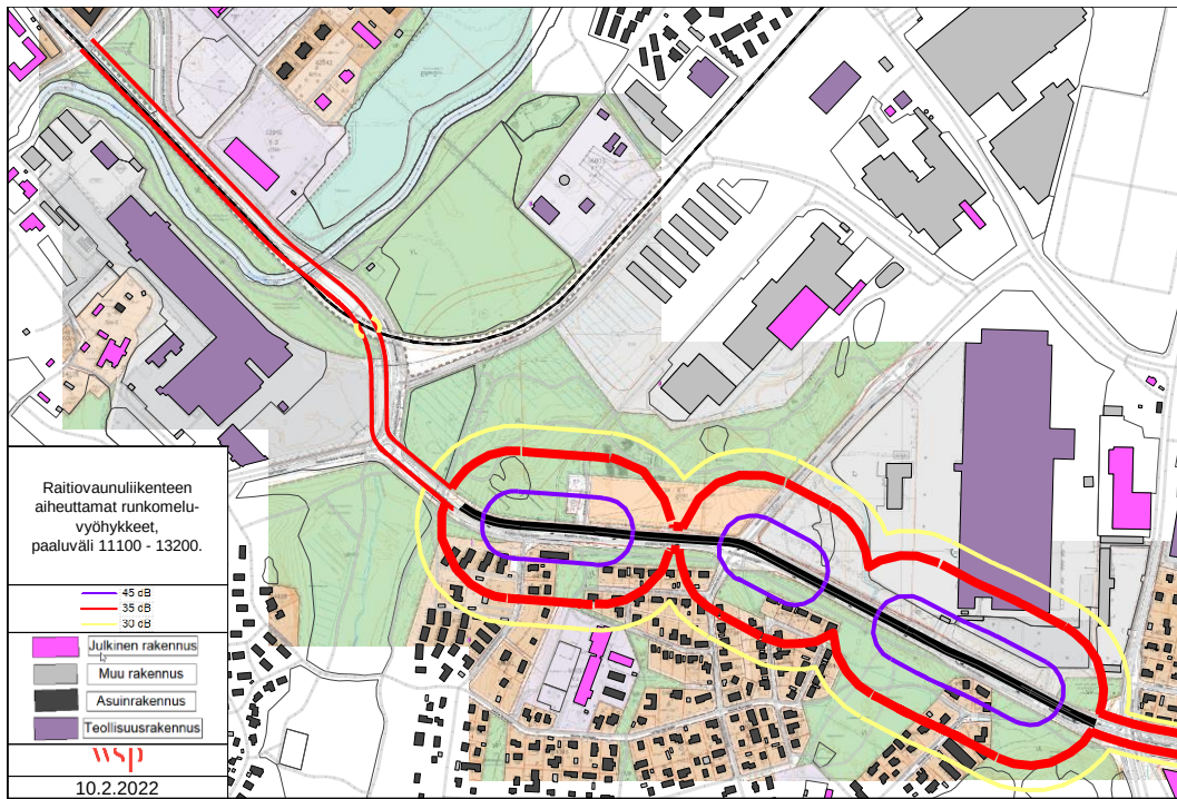
Kuva 6. Raitiovaunuliikenteen aiheuttamat runkomelualueet Kuninkaalan alueella, paaluväli 11100 – 13200.
