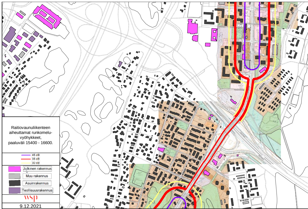
Kuva 8. Raitiovaunuliikenteen aiheuttamat runkomelualueet Hakunilan eteläosassa ja Vaaralan pohjoisosissa, paaluväli 15400 - 16600.
