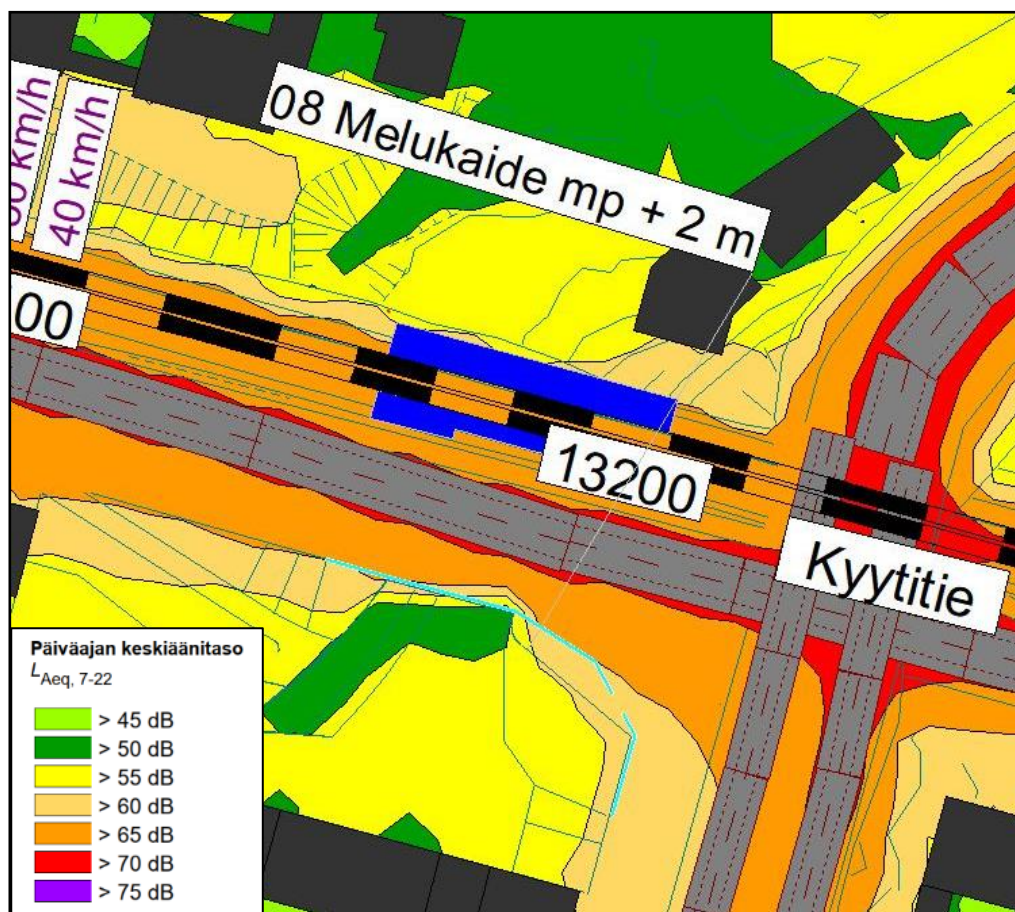
Kuva 10 "Valoaukion" suojaksi esitetään 2 m korkea (maanpinnasta) melukaidetta ääniympäristön parantamiseksi.
