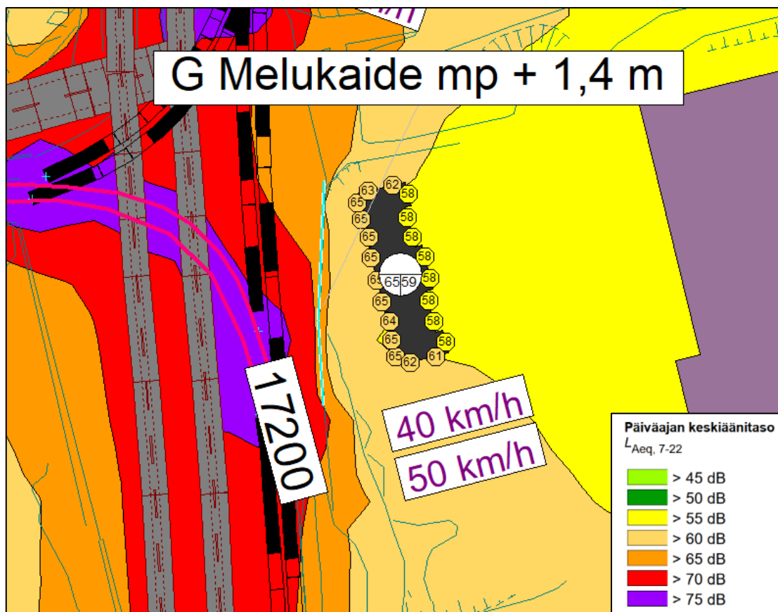
Kuva 16 Julkisivua suojaava melukaide G paalulla 17150.
