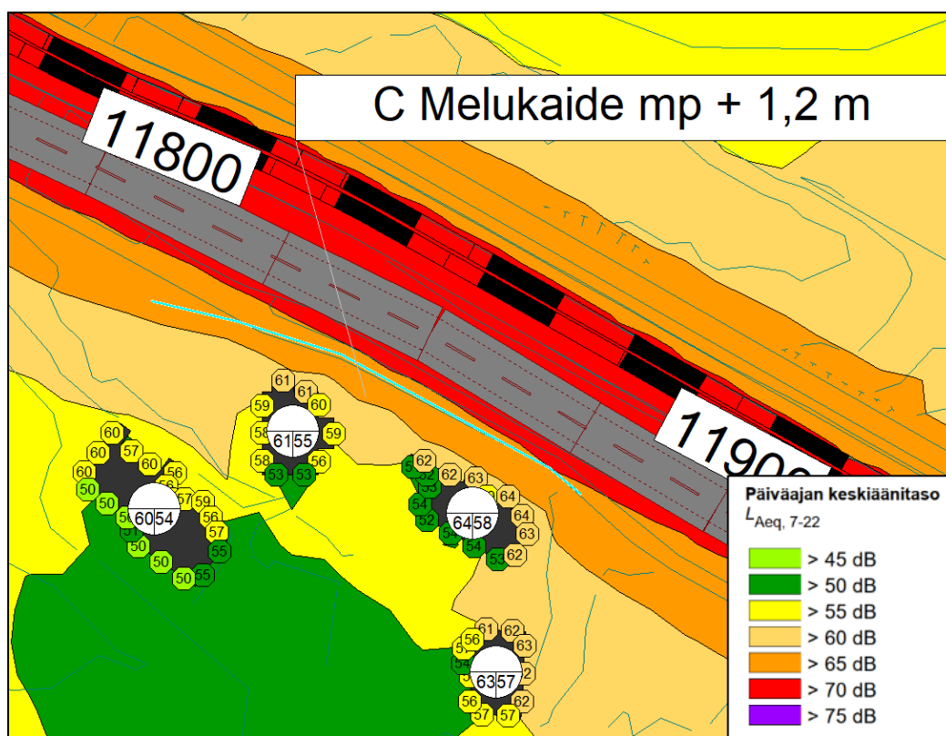
Kuva 8 Julkisivuja suojaava melukaide C paaluvälillä noin 11800–11900.
