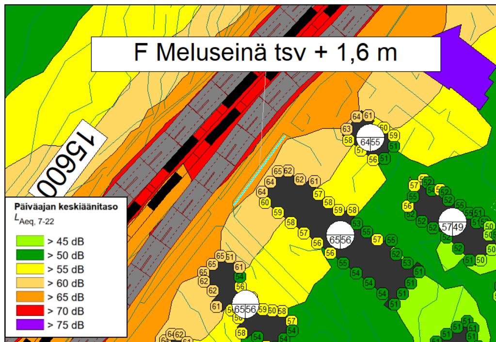
Kuva 14 Julkisivua suojaava 1,6 m korkea ja 24 m metriä pitkä meluseinä
