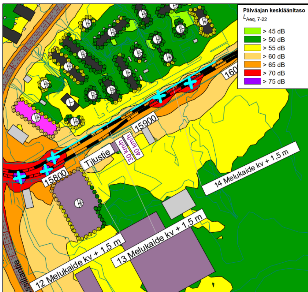
Kuva 15 Tilustien tarkasteltu meluntorjunta, 1,5 m korkeat melukaiteet torjuvat oleskelualueet pöösosin ohjearvojen alapuolelle.
