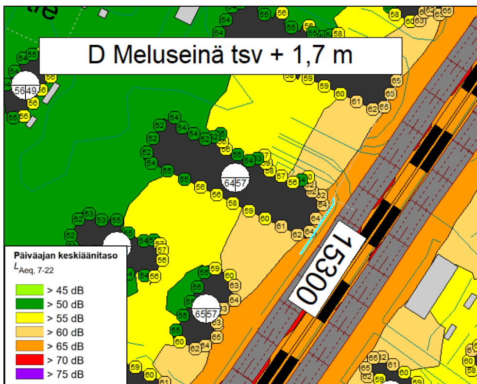
Kuva 12 Julkisivua suojaava 1,7 m korkea ja 18 metriä pitkä meluseinä D paalulla 15300.
