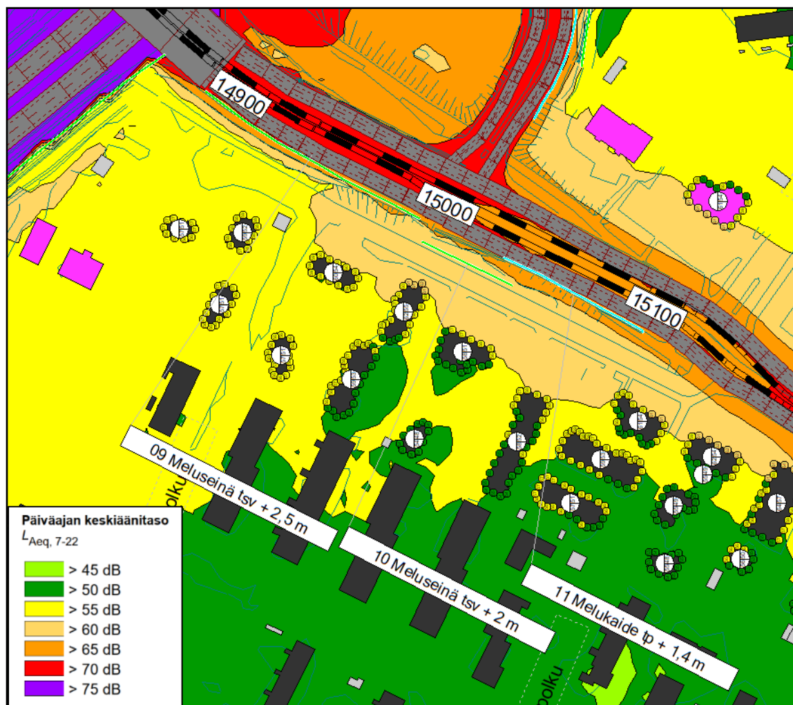
Kuva 11 Hakunilantien tarkasteltu meluntorjunta paaluvälillä 14900–15100.
