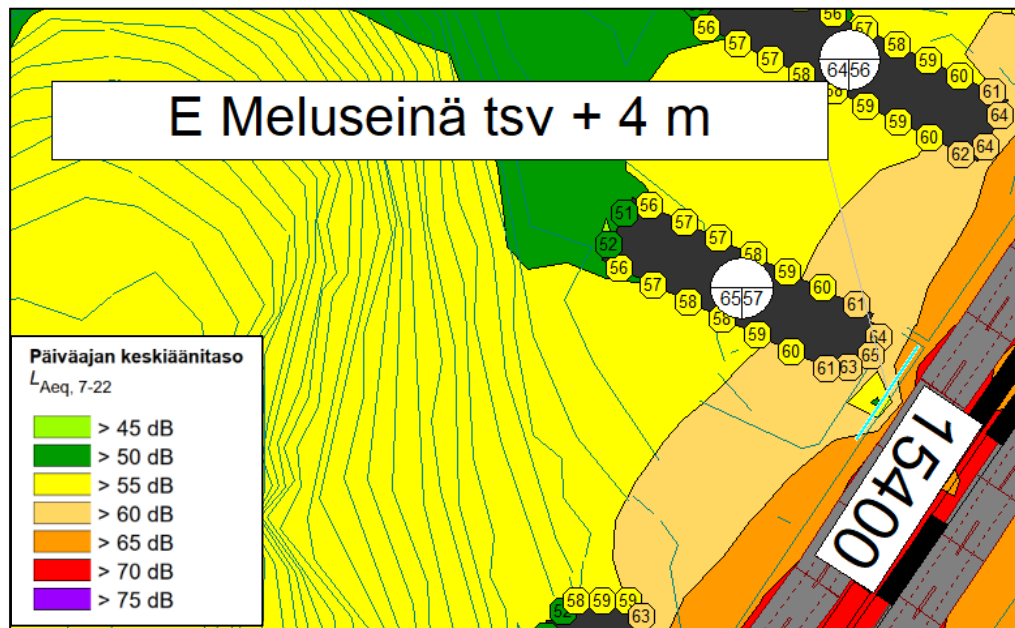
Kuva 13 Julkisivua suojaava 4 m korkea ja 14 m metriä pitkä meluseinä E paalulla 15400.
